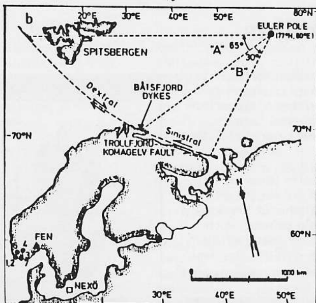
Kuva 2: Paleomagneettisista mittauksista konstruoidut mallit siirroksen suunnalle ja suuruudelle. Lähde: LJ Pesonen, TH Thorsvik, SÅ Elming & Bylund 1988; Crustal evolution of Fennoscandia - paleomagnetic constraints
