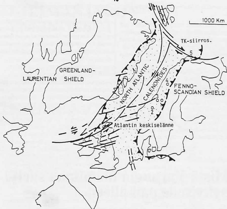
Kuva 1: Kaavakuva Pohjois-Atlantin aukeamisesta.
